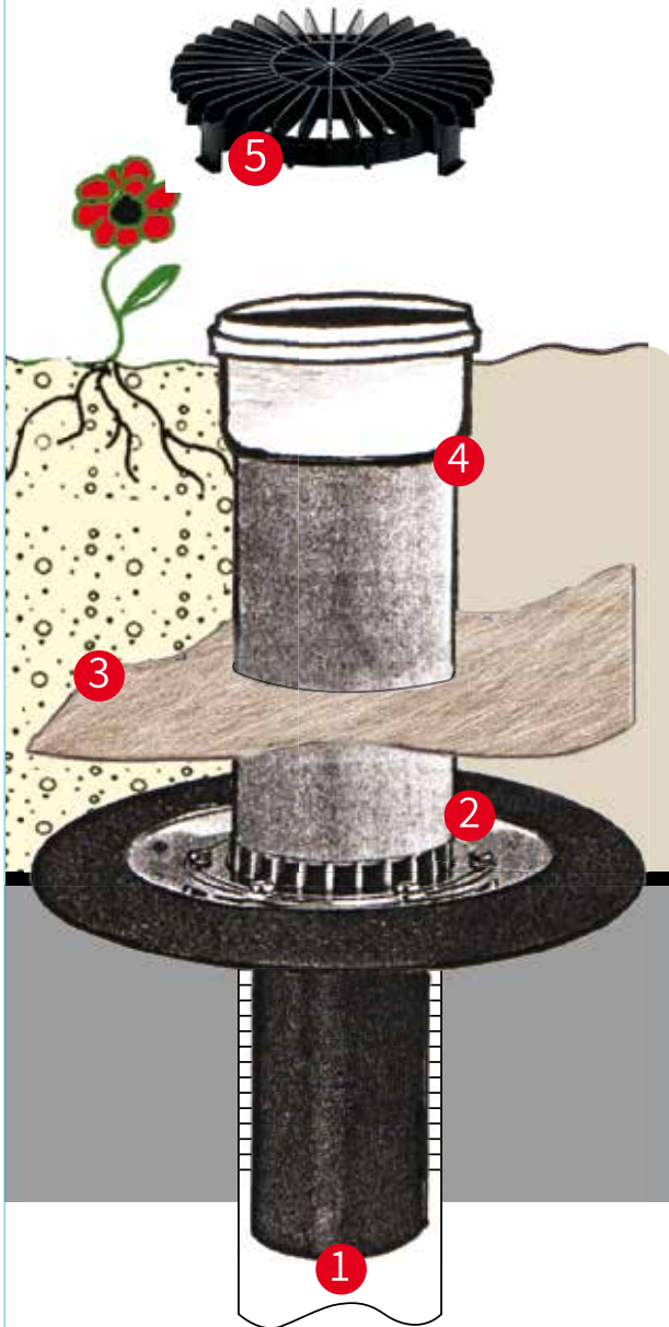
מבנה האביזרים S-15 בניקוז אדנית (ערוגה) צמחיה.
